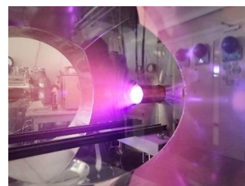
図 4 原子状酸素照射試験
